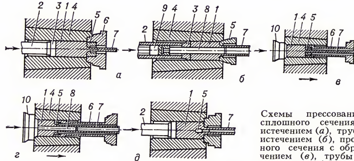
Схемы прессования профиля сплошного сечения (прессование со сваркой, д ); 1 — заготовка; 2 — пресс-штемпель; 3 — пресс-шайба; 4 — контейнер; 5 — матрица; 6 — матрицедержатель; 7 — пресс-изделие; 8 — игла; 9 — иглодержатель; 10 — пробка.
